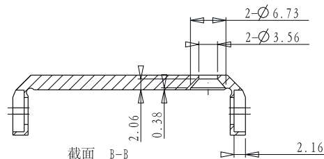
截面 B-B
